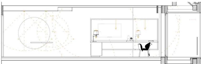
Elévation Est 1:50
